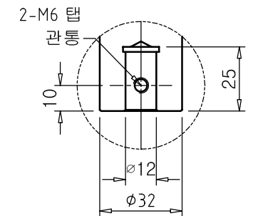
상크롤 상세도
